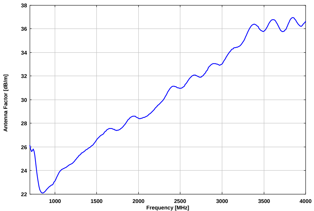
Antennenfaktor (k-Faktor):
